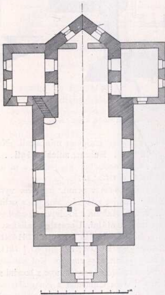
Obr. 371. Velké Chrastice. Půdorys kostela.
